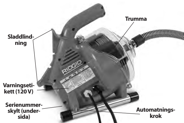
Figur 2 – PowerClear avloppsrensmaskin
