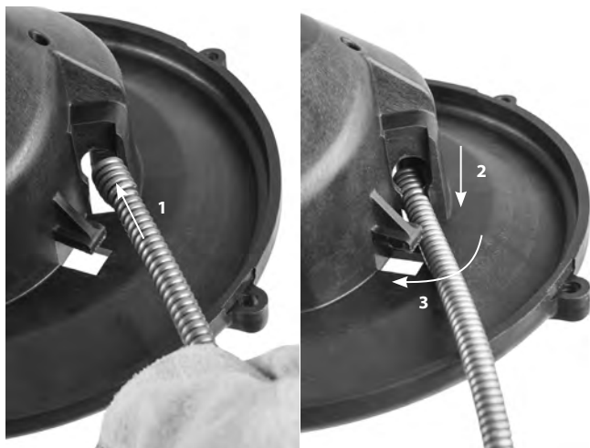
Slika 15 – Pritrjevanje kabla v notranji bobnen
