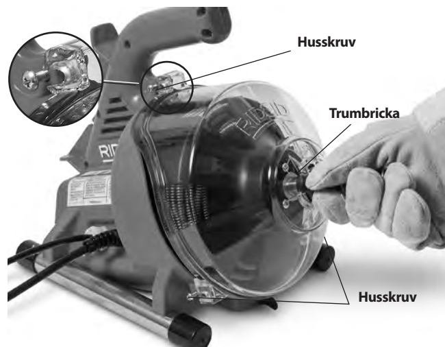
Figur 13 – Öppna avloppsrensaren
