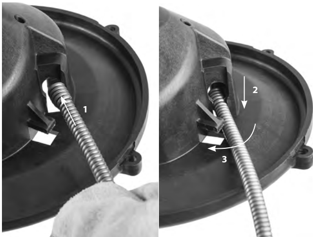
15. ábra – A kábel rögzítése a dob belső részéhez
