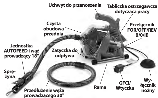
Rysunek 1 - Maszyna do czyszczenia odpływów PowerClear
