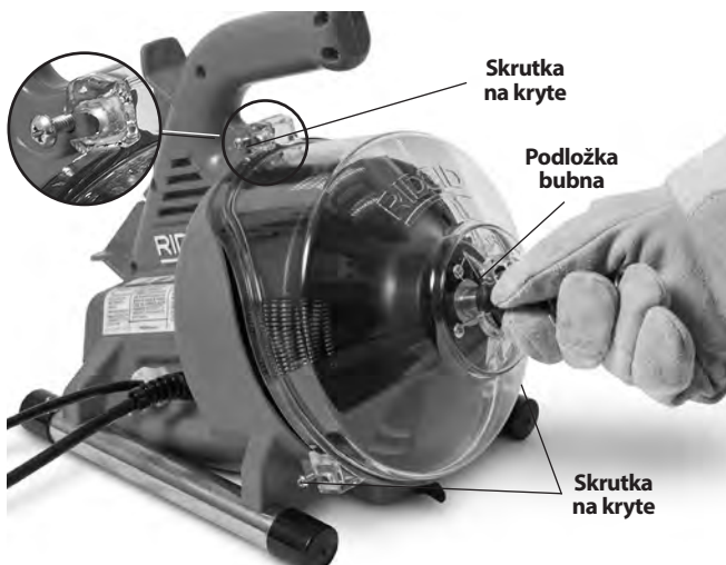
Obrázok 13 – Otvorenie čističky odtokov
